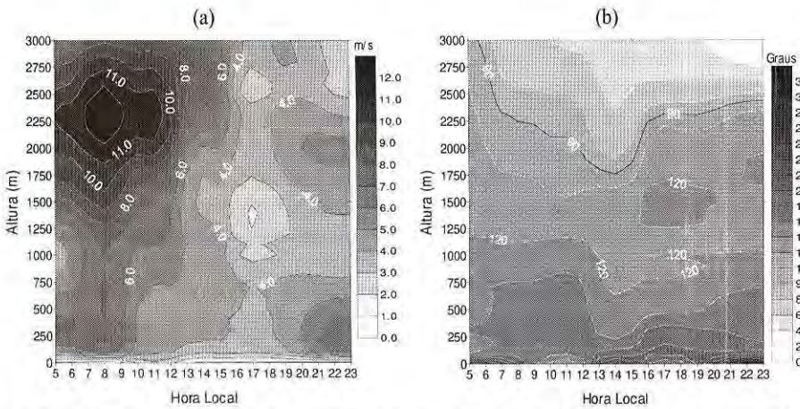
Figura 7. Evolução Temporal do Vento na Pastagem no dia 15 : Velocidade (a) e Direção (b)
