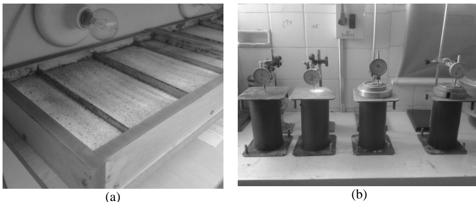
Figura 3 - (a) Ensaio de avaliação da fissuração e perda de água; e (b) Ensaio de avaliação das retrações linear livre e comprimida por meio de secagem natural
