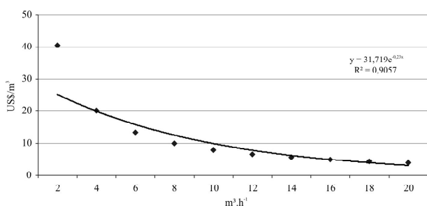
Figura 3 – Comportamento do custo de extração de madeira, em função do rendimento operacional.
