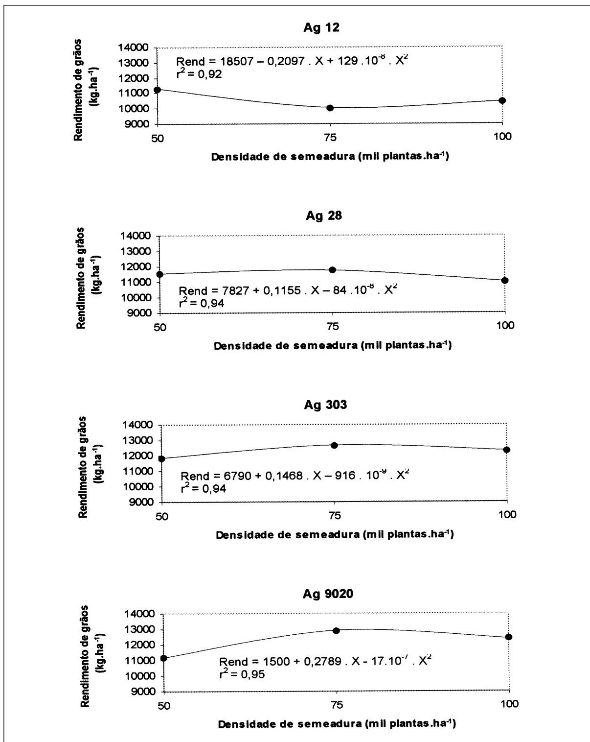
Figura 1 - Rendimento de grãos de híbridos de milho das décadas de 60 (Ag 12), 70 (Ag 28), 80 (Ag 303) e 90 (Ag 9012) em diferentes densidades de sementeira. Lages, SC, 1999/2000.
