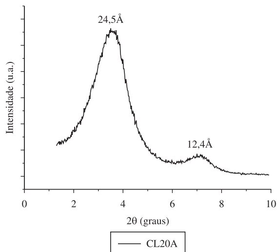
Figura 5. Difratoograma de raios-X da argila organofílica CL20A.
