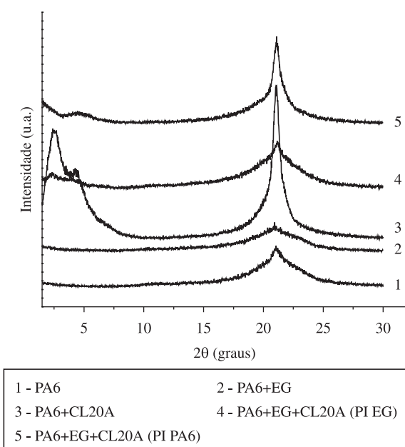
Figura 6. Difratoogramas de raios-X da PA6 e dos sistemas.
