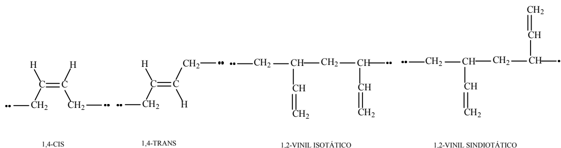
Figura 1. Estruturas butadiênicas
