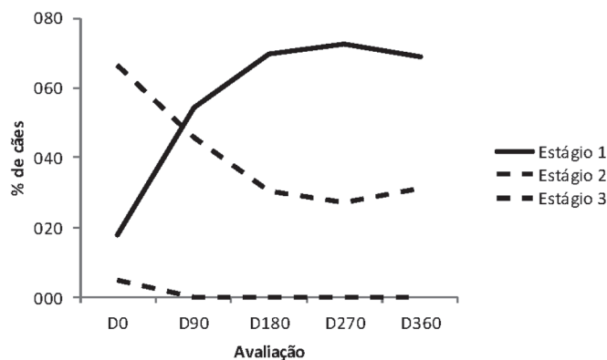
Fig.1. Evolução do estadiamento clínico dos cães atendidos no Hospemv-UFBA entre 2012-2014, naturalmente infectados por Leishmania infantum e tratados contra leishmaniose visceral. Os cães foram agrupados conforme as avaliações realizadas no D0, D90, D180, D270 e D360 e o resultado foi expresso em percentual de cães que foram categorizados em estágio 1 (cães sem doença clínica/doença clínica branda, com anemia e proteína total normal ou alterada); estágio 2 (cães sem doença clínica /com doença clínica branda, sem ou com anemia e com proteína total alterada, estágio 3 (cães com doença severa, com anemia e com proteína total alterada)
