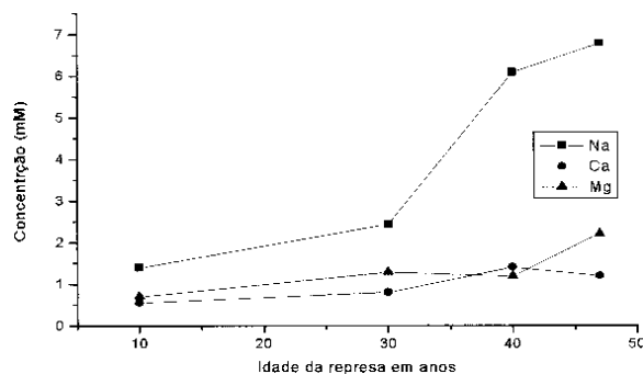
Figura 3. Variação da concentração de sódio, cálcio e magnésio em represas (Angico, Divino, Tremedal e Anajé) de demanda irregular construídas em épocas diferentes.
