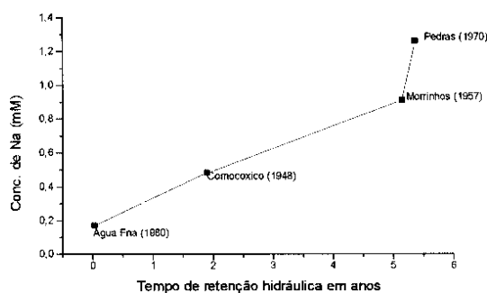
Figura 4. Variação da concentração do sódio em relação ao tempo de retenção das represas (Comocoxico, Morrinhos, Pedras e Água Fria) de demanda regulares.
