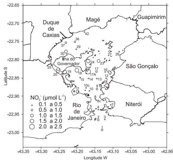
Figura 2. Distribuição espacial das concentrações de nitrito (NO 2 - ) em águas superficiais nas 37 estações amostradas na Baía de Guanabara no período de 5 a 7 de abril de 2004
