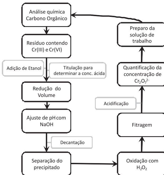
Figura 1. Fluxograma do procedimento de reciclagem do resíduo contendo crômio
