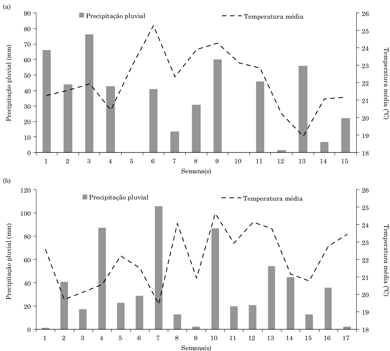
Figura 1. Precipitações pluviométricas e temperaturas médias referentes aos períodos experimentais das safras da seca - 2012 (a) e das águas - 2012/2013 (b). Estação experimental do Iapar, Ponta Grossa, PR.
