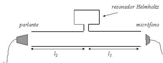
Figura 1. Resonador Helmholtz insertado lateralmente en un tubo abierto en ambos extremos.
