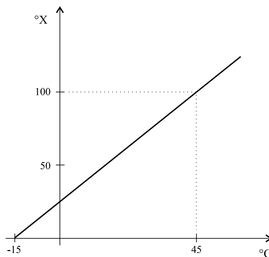
Figura 1 - Temperatura em dois termômetros: em °X e °C.
