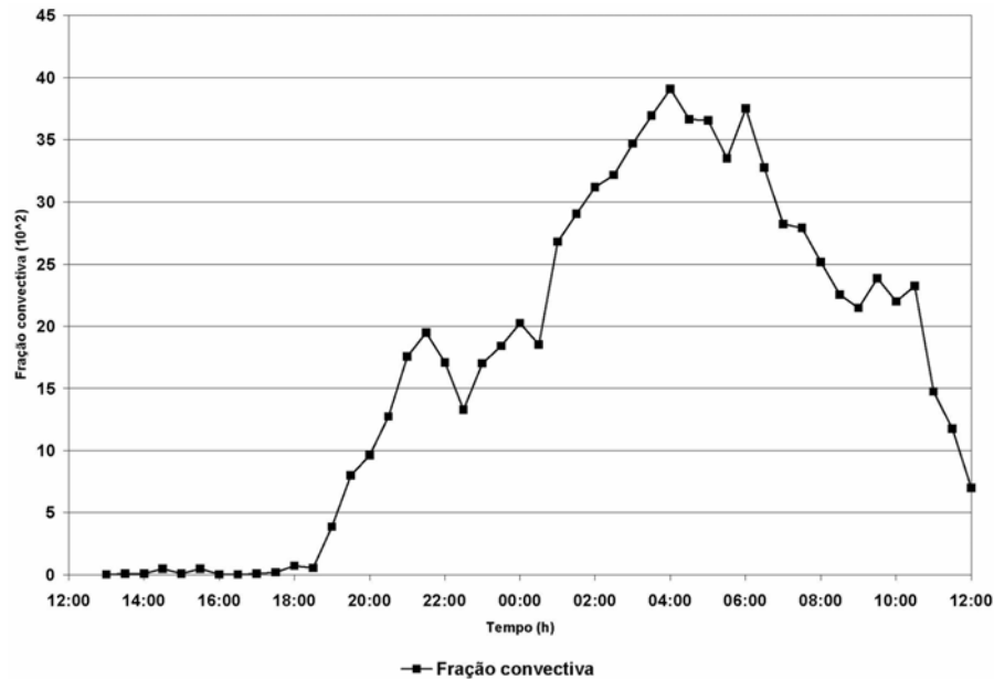
Figura 4 – Evolução temporal da fração convectiva (estimada via satélite) do SCM que atingiu o estado do Rio Grande do Sul, entre as 12 UTC do dia 19/02/03 e as 12 UTC do dia 20/02/03.
