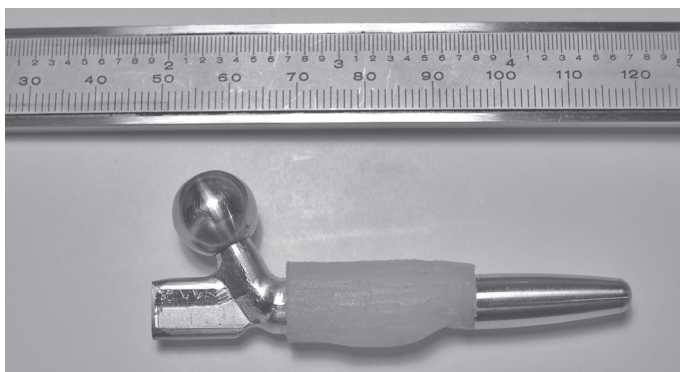
Figura 3 – Configuração final do implante após a sua maquinagem.
