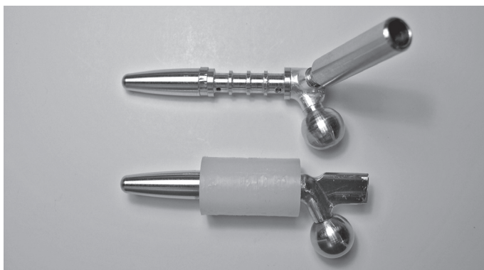
Figura 2 – Na parte superior, o modelo mestre fabricado para receber o polivinilsiloxano. Na parte inferior a pré-prótese preparada para ser maquinada com a geometria do canal femoral.
