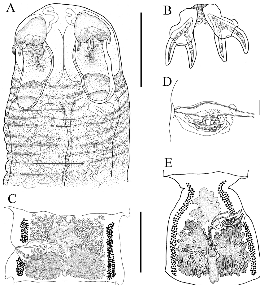
Figure 2. Acanthobothrium marquesi n. sp. A. Scolex. B. Hooks. C. Mature proglotid. D. Cirrus sack. E. Terminal proglotid. Scale bar: A. 750 \mu m; B. 150 \mu m; C. 1000 \mu m; D. 133 \mu m; E. 880 \mu m.
