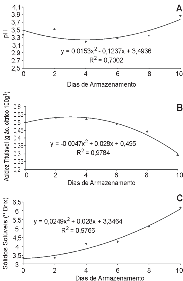
Figura 4. pH, acidez titulável e sólidos solúveis da polpa de mangas 'Palmer' revestidas por fécula de mandioca preparada com água de cravo ou de canela, armazenadas por 10 dias.
