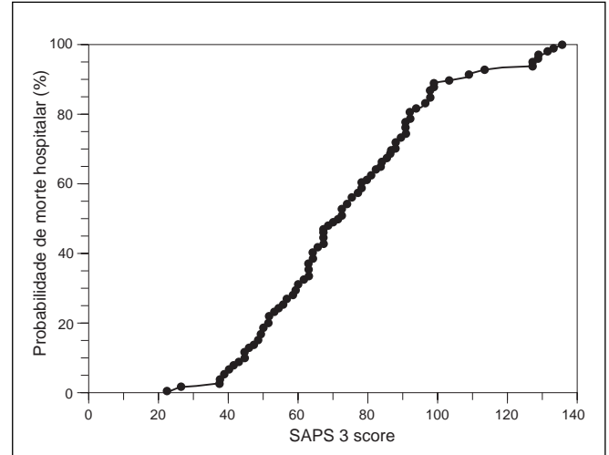
Figura 3 – Relação entre o sistema SAPS 3 e a probabilidade de morte hospitalar. A probabilidade de morte hospitalar dos pacientes aumenta consideravelmente conforme maior a pontuação encontrada do escore SAPS 3.
