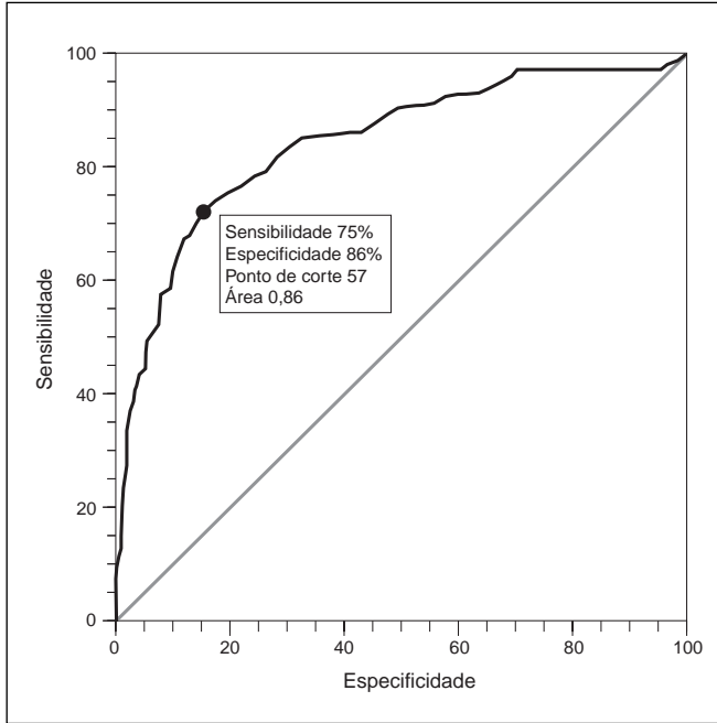
Figura 1 – Curva ROC do SAPS 3 na predição de mortalidade hospitalar. O valor de 57 apresentou melhor sensibilidade (75%) e especificidade (86%) para mortalidade hospitalar, com área sob a curva de 0,86 (Área = 0,5; p < 0,001 , IC95%; 0,83-0,88)
