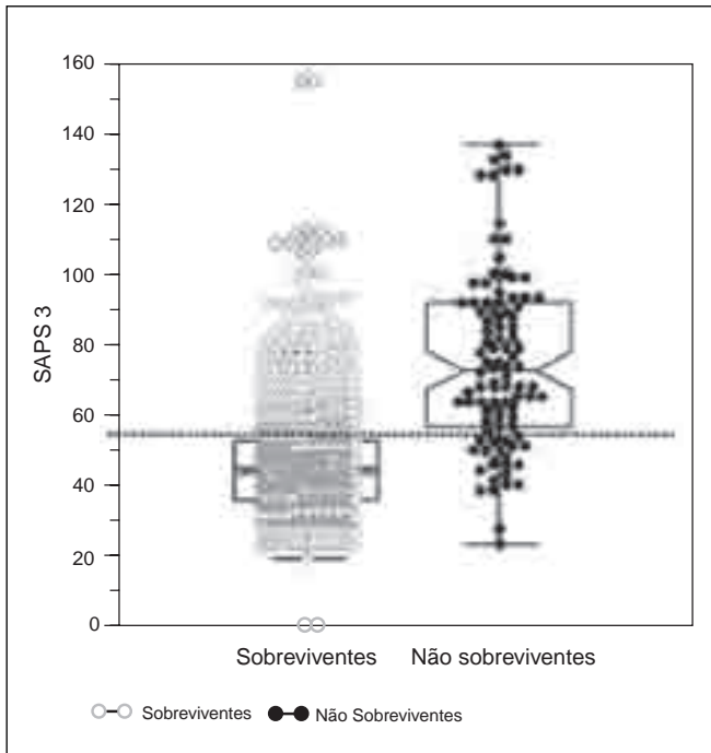
Figura 2 – Distribuição dos pacientes relacionando o escore e a evolução dos mesmos (p) Dos pacientes com índice SAPS 3 maior a 57, 73,5% não sobreviveram versus 26,5% de sobreviventes (OR = 1,32 IC 95% 1,23-1,42, p < 0,0001 ).
