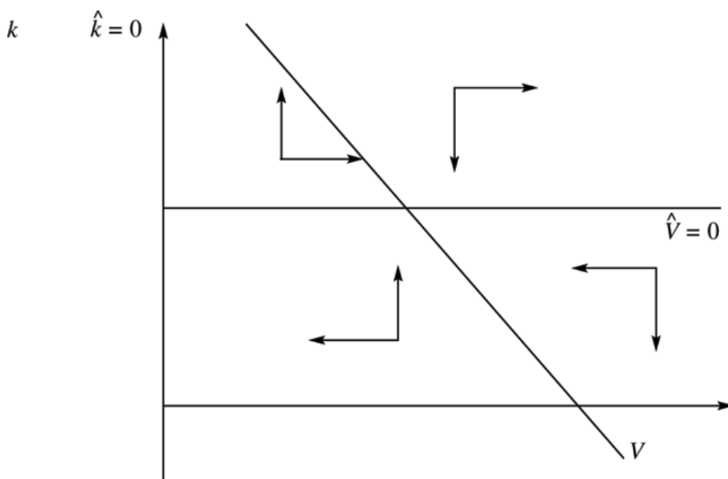
Figura 1: Equilíbrio Estável
