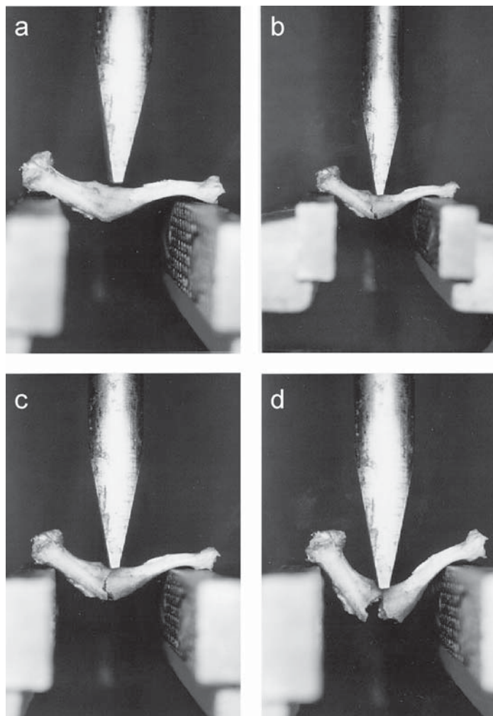
Figura 5 (a-d) - Tibia, com fratura, montada na máquina universal de ensaio. Seqüência do ensaio de flexão até a ruptura do corpo de prova.
