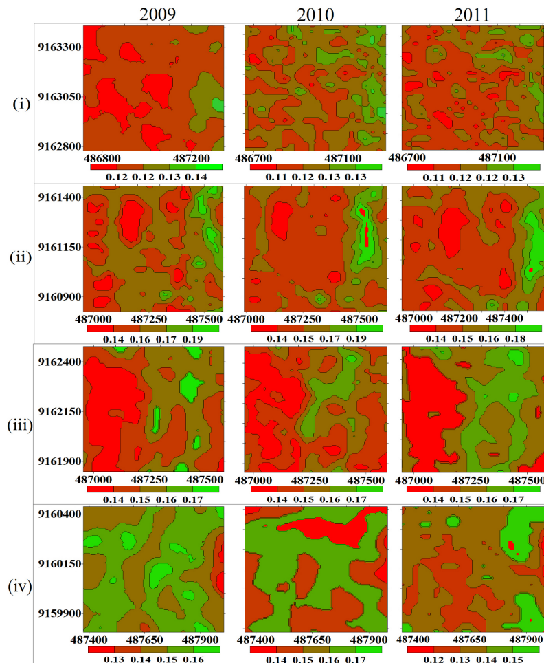
Figura 04 - Albedo de (i) Floresta Amazônica Natural; (ii) Floresta Amazônica Manejada; (iii) Sistema Silvistoril, e; (iv) Pastagem ( Brachiaria brizantha ).
