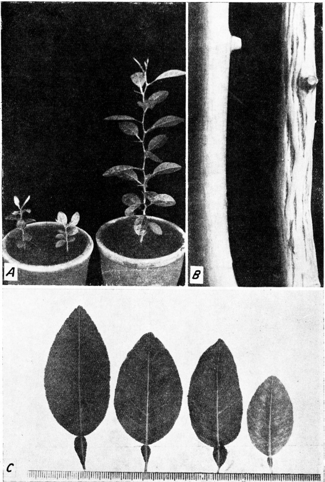
Teste do limão galego. A — Plantas de pé franco da mesma idade inoculadas por afídios virulíferos (esquerda) e testemunha. B — Galhos descascados de planta sadia (esquerda) e de planta com tristeza mostrando "pitting" no lenho. C — Fôlhas de planta com tristeza mostrando palidez das nervuras e de planta sadia (à esquerda).
