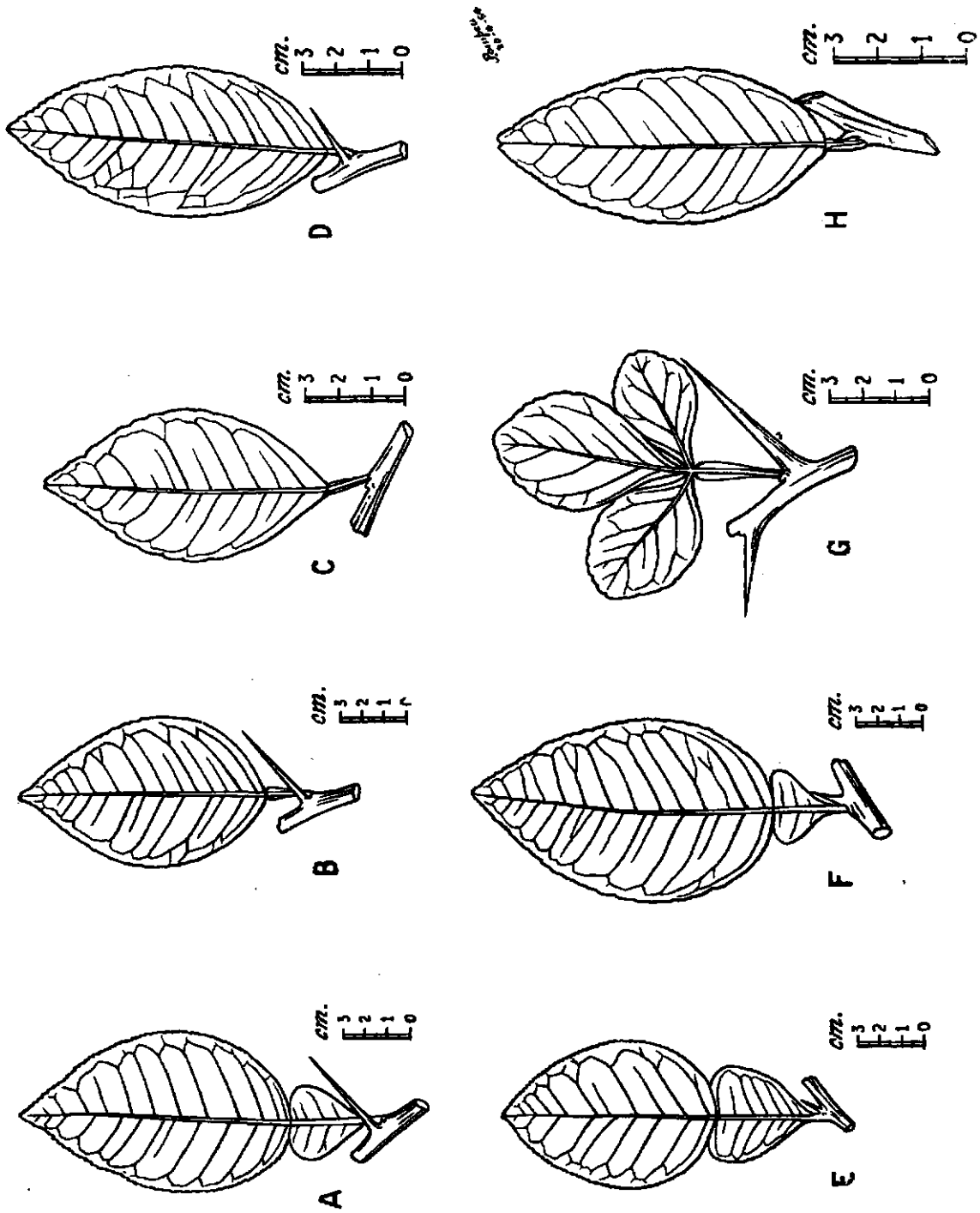
FIGURA 1. — Fôlhas, pecíolos e espinhos das principais espécies cítricas: A — laranja azêda; B — laranja doce; C — tangerina; D — limão; E — toranja; F — pomelo; G — trifoliata; H — limão cravo (Rangpur).
