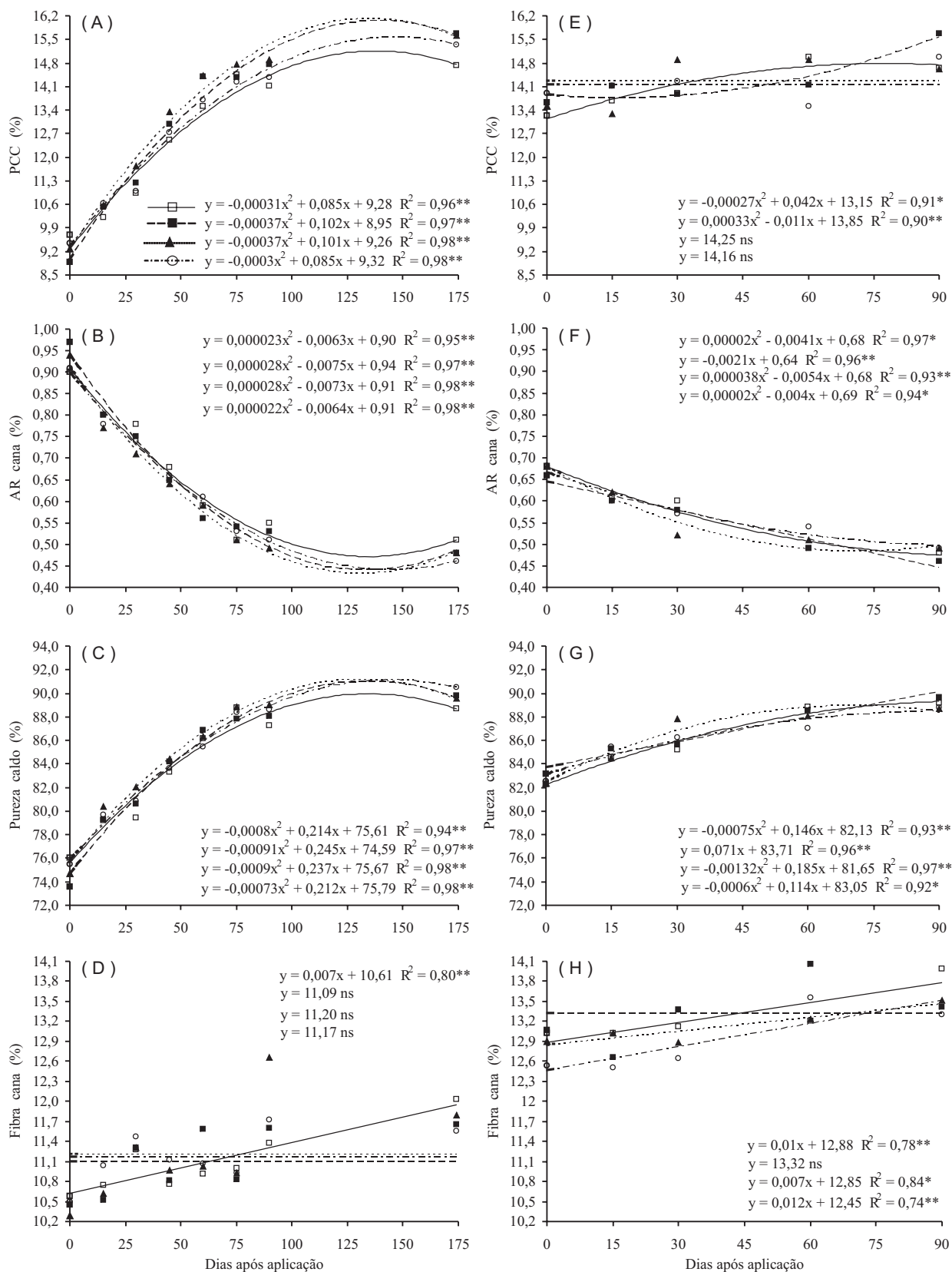
Figura 2. PCC da cana (%), AR na cana (%), Pureza do caldo (%) e Fibra na cana (%) em função da aplicação dos tratamentos testemunha ( \square ), Sulfometuron metil ( \blacksquare ), Glifosato ( \blacktriangle ) e C.C. + Glifosato ( \circ ) na variedade de cana-de-açúcar SP80-3280, Igarçu do Tietê, SP, na safra 2004 (A, B, C, D) e na safra 2005 (E, F, G, H). ns: Não significativo. * e **: Significativo pelo teste F, respectivamente, a 5% e 1% de probabilidade.
