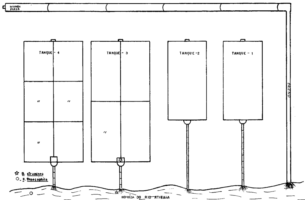
Fig. 8 — Planta esquemática do Posto Experimental de Biologia e Piscicultura de Americana, Estado de São Paulo.
