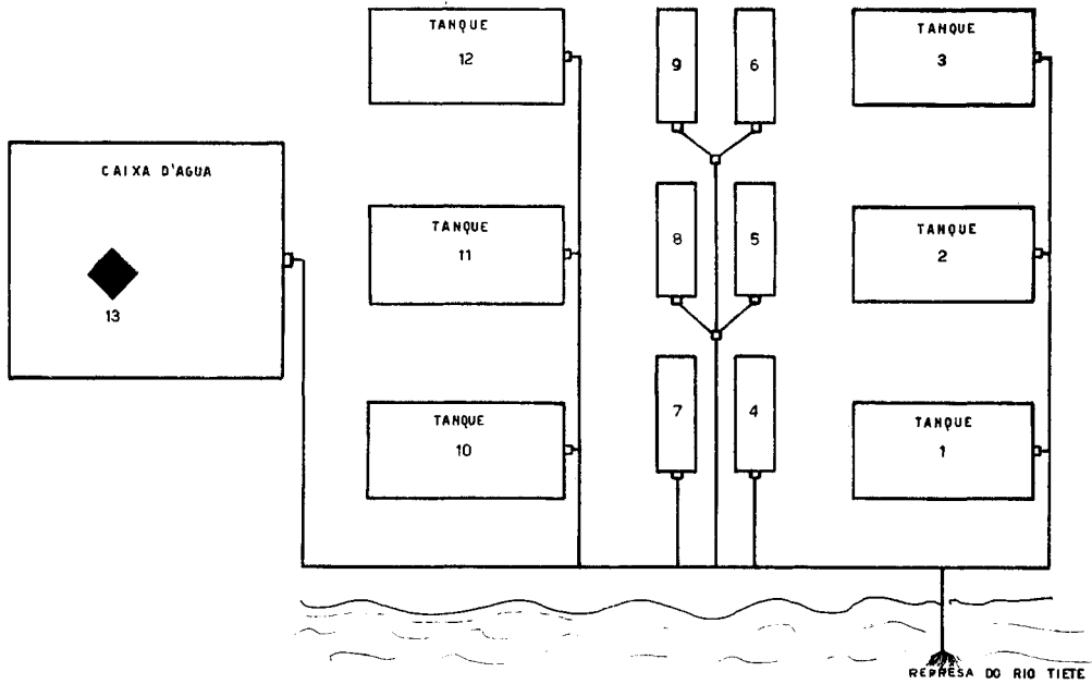
Fig. 6 — Planta esquemática da Estação Experimental de Biologia e Piscicultura de Barra Bonita, Estado de São Paulo. Campanha de Combate à Esquistossomose — Foco de Biomphalaria straminea .
