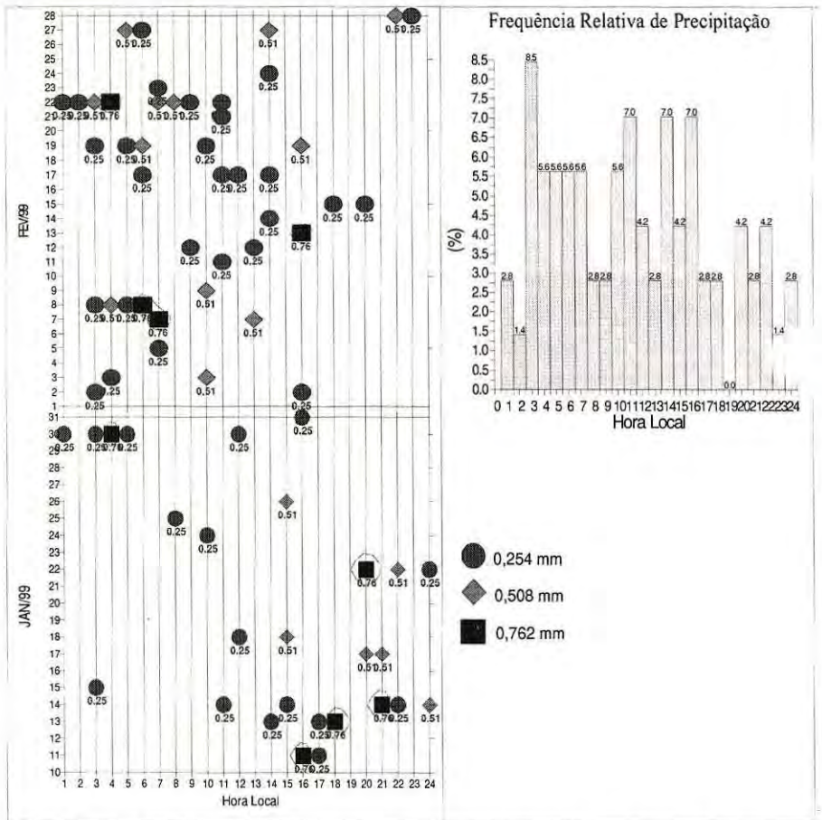
Figura 4. Série Temporal e Frequência Relativa da Precipitação inferior a 1 \text{ mm.h}^{-1} .
