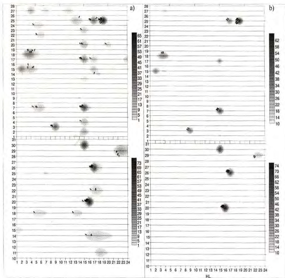
Figura 6. Série temporal e frequência relativa de precipitação superior à 1 mm.h -1 (a) e 10 mm.h -1 (b).
