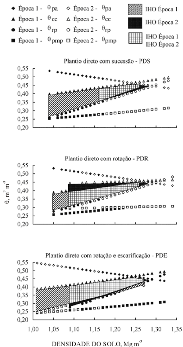
Figura 1. Variação do conteúdo de água ( \theta ) com a densidade do solo para os três tratamentos, nos níveis críticos de capacidade de campo ( \theta_{cc} ), ponto de murcha permanente ( \theta_{pmp} ), porosidade de aeração de 0,10 m 3 m -3 ( \theta_{pa} ) e resistência do solo à penetração de 3,5 MPa ( \theta_{rp} ). Áreas hachuradas correspondem ao intervalo hídrico ótimo (IHO) nas épocas de amostragem.
