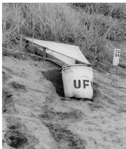
Figura 2. Sistema coletor da suspensão de água + solo escoado.
