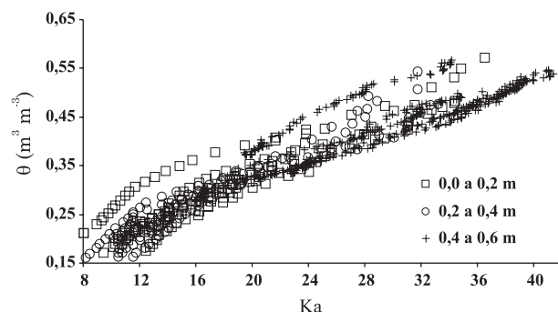
Figura 1. Valores de umidade do solo com base em volume, \theta , e de K_a , em diferentes valores de densidade do solo, obtidos nas três camadas de solo estudadas.
