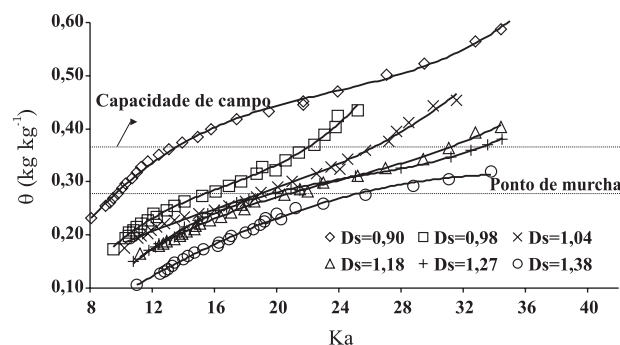
Figura 2. Valores de umidade do solo com base em massa, \theta_g , e de K_a em diferentes valores de D_s ( Mg m^{-3} ), obtidos nas três camadas de solo estudadas.
