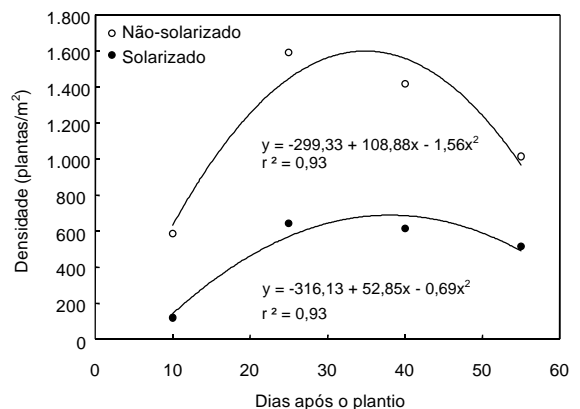
FIG. 1. Efeito da solarização do solo na reinfestação de tiririca ( Cyperus rotundus ) em cultivos orgânicos de hortaliças, segundo a época de amostragem (Seropédica, RJ, 1998).
