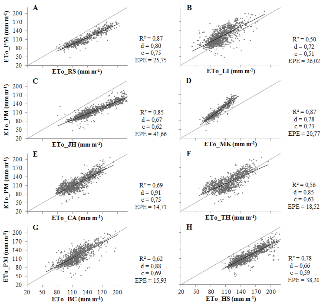
FIGURA 3 - Evapotranspiração de referência na escala mensal (ETo, mm m -1 ), estimado pelo método de Penman-Monteith (ETo PM ), em relação aos métodos de Radiação Solar (ETo RS ) (A), Linacre (ETo LI ) (B), Jensen-Haise (ETo JH ) (C), Makkink (ETo MK ) (D), Camargo (ETo CA ) (E), Thornthwaite (ETo TH ) (F), Blaney-Criddle (ETo BC ) (G) e Hargreaves-Samani (ETo HS ) (H), para o período de outubro a março, nos anos de 1961 a 2010, na região da Campanha-RS. Índice de determinação (R 2 ), de exatidão (d), de desempenho (c) e Erro-Padrão da Estimativa (EPE, mm m -1 ).
