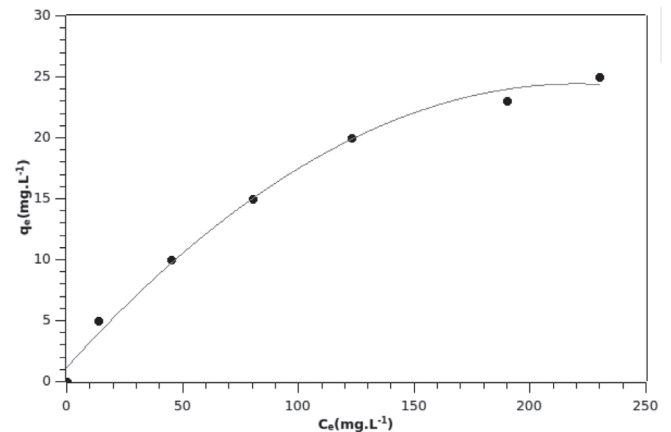
Figura 4. Exemplo de isoterma de adsorção. Adaptada da ref. 33
