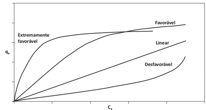
Figura 5. Comportamentos possíveis para isotermas de adsorção 33
