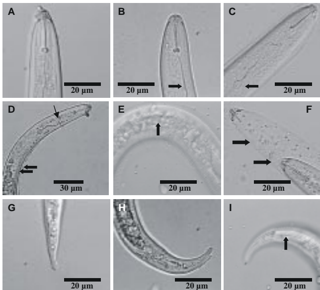
FIG. 4 - Fotomicrografias de fêmeas jovens de Rotylenchulus reniformis . A) Região labial cônica. B) Região labial arredondada e abertura da glândula dorsal esofagiana (seta). C) Metacorpo com válvula esclerotizada (seta). D) Sobreposição ventral do esôfago sobre o intestino (setas) e abertura da glândula dorsal esofagiana (seta). E) Campo lateral com quatro incisuras (seta). F) Cutículas remanescentes de duas ecdises anteriores (setas). G e H) Variações na forma da cauda. I) Fasmídio (seta).
