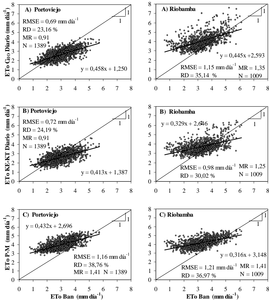
FIGURA 3. Evapotranspiración de referencia ( ETo ) estimada para un periodo móvil de tres días, obtenida con los modelos de: A) C_{HO} Diario (Holdridge), B) KE-KT Diario (H-S) y C) Penman-Monteith (P-M) en una representación 1:1, comparada con ETo Ban durante el periodo 2000-2005 para Portoviejo (costa) y Riobamba (Región Andina). Reference evapotranspiration ( ETo ) estimated for a mobile period of three days, using the models: A) C_{CHO} daily (Holdridge), B) KE-KT daily (H-S) and C) Penman-Monteith (P-M) in a 1:1 representation, compared with ETo Pan during the 2000-2005 period for Portoviejo (coast) and Riobamba (Andes region).
