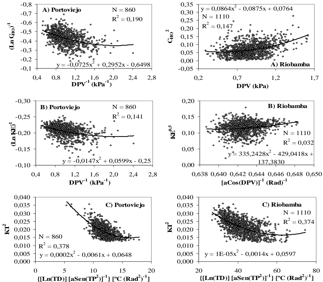
FIGURA 1. Coeficientes diarios A) C_{HO} (Holdridge) y B) KE (H-S) en función del déficit de presión de vapor diario (DPV), y C) KT (H-S) en función de la temperatura media diaria (TP) y la amplitud térmica diaria (TD) para Portoviejo (costa) y Riobamba (Región Andina). Daily coefficients A) CHO (Holdridge) and B) KE (H-S) as a function of vapor pressure deficit (DPV), and C) KT (H-S) as a function of daily average temperature (TP) and daily amplitude of the air temperature (TD) for Portoviejo (coast) and Riobamba (Andes region).
