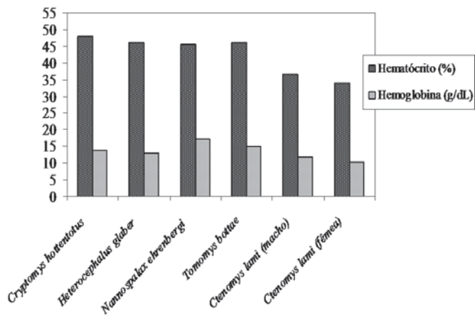
Fig.2. Comparação entre os valores médios de Hematócrito (%) e Hemoglobina (g/dL) de diferentes espécies de roedores subterrâneos com a espécie de roedor subterrâneo Ctenomys lami . Fontes: Buffenstein (2000), Johansen et al. (1976), Lechner (1976), Arieli & Shkolnik (1977).
