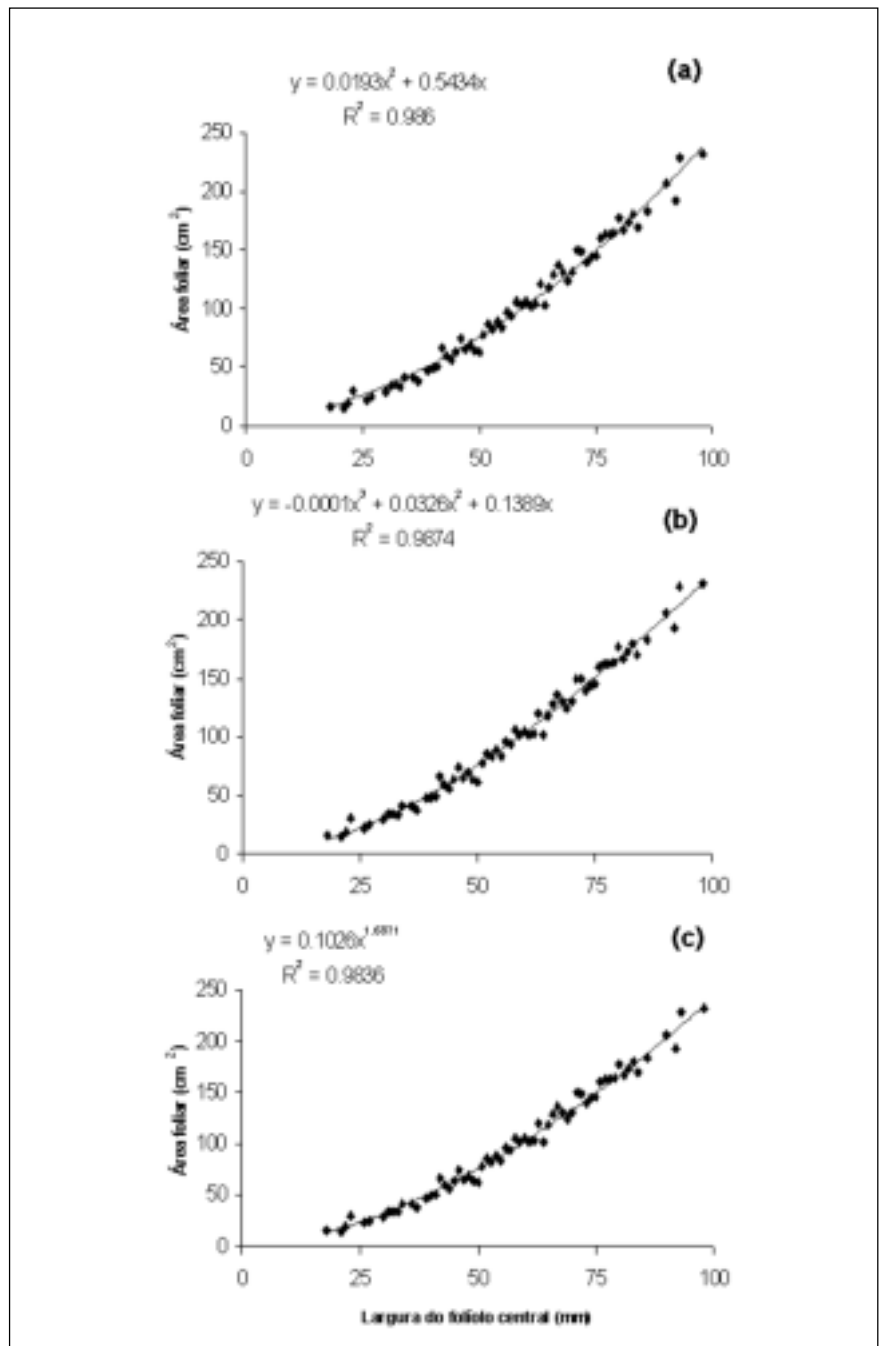
Figura 1. Curvas de regressão não-linear (a-quadrática, b-cúbica e c-potência) obtidas entre a largura máxima do folíolo central e a área foliar total da folha, utilizando o medidor de área foliar, em plantas de feijão-vagem. Londrina, UEL, 1999.
