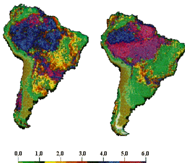
Figura 7 - Índice de Área Foliar da América do Sul: a) janeiro e b) julho. (Fonte: Myneni et al., 1997).
