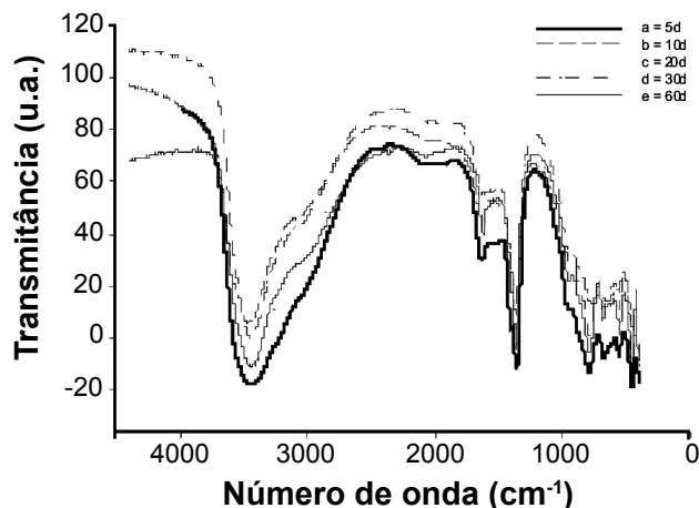
Figura 7: Espectros de infravermelho para os compostos sintetizados no experimento 3: a) HDL LV-23, b) HDL LV-22, c) HDL LV-21, d) HDL LV-20 e e) HDL LV-19.
