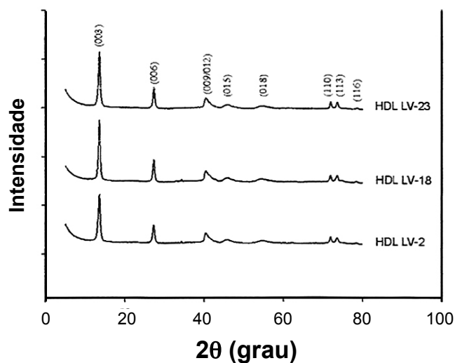
Figura 1: Difratogramas de raios X dos compostos sintetizados no experimento 1 (HDL LV-2), experimento 2 (HDL LV-18) e experimento 3 (HDL LV-23).
