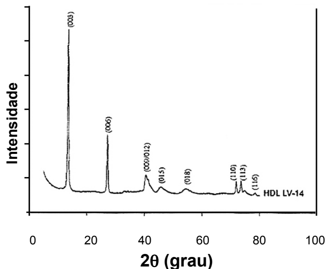
Figura 2: Difratogramas de raios X do composto sintetizado no experimento 2 (HDL LV-14).
