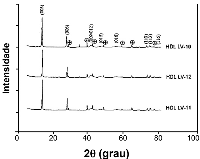
Figura 3: Difratogramas de raios X dos compostos sintetizados no experimento 1 (HDL LV-11), experimento 2 (HDL LV-12), experimento 3 (HDL LV-19) e \oplus hematita.
