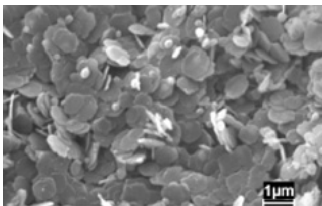
Figura 10: Imagem de microscopia eletrônica de varredura do composto HDL LV-20.
