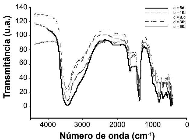
Figura 5: Espectros de infravermelho para os compostos sintetizados no experimento 1: a) HDL LV-2, b) HDL LV-10, c) HDL LV-3, d) HDL LV-13 e e) HDL LV-11.
