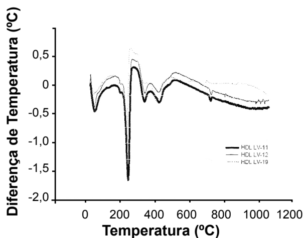
Figura 8: Curvas de análise térmica diferencial das amostras HDL LV-11, HDL LV-12 e HDL LV-19.
