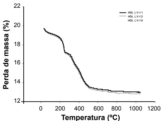
Figura 9: Curvas de análise termogravimétrica das amostras HDL LV-11, HDL LV-12 e HDL LV-19.
