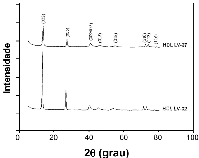
Figura 4: Difratogramas de raios X dos compostos sintetizados a pH 9 (HDL LV-37) e razão 4 (HDL LV-32).
