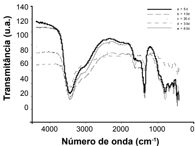
Figura 6: Espectros de infravermelho para os compostos sintetizados no experimento 2: a) HDL LV-18, b) HDL LV-16, c) HDL LV-15, d) HDL LV-14 e e) HDL LV-12.
