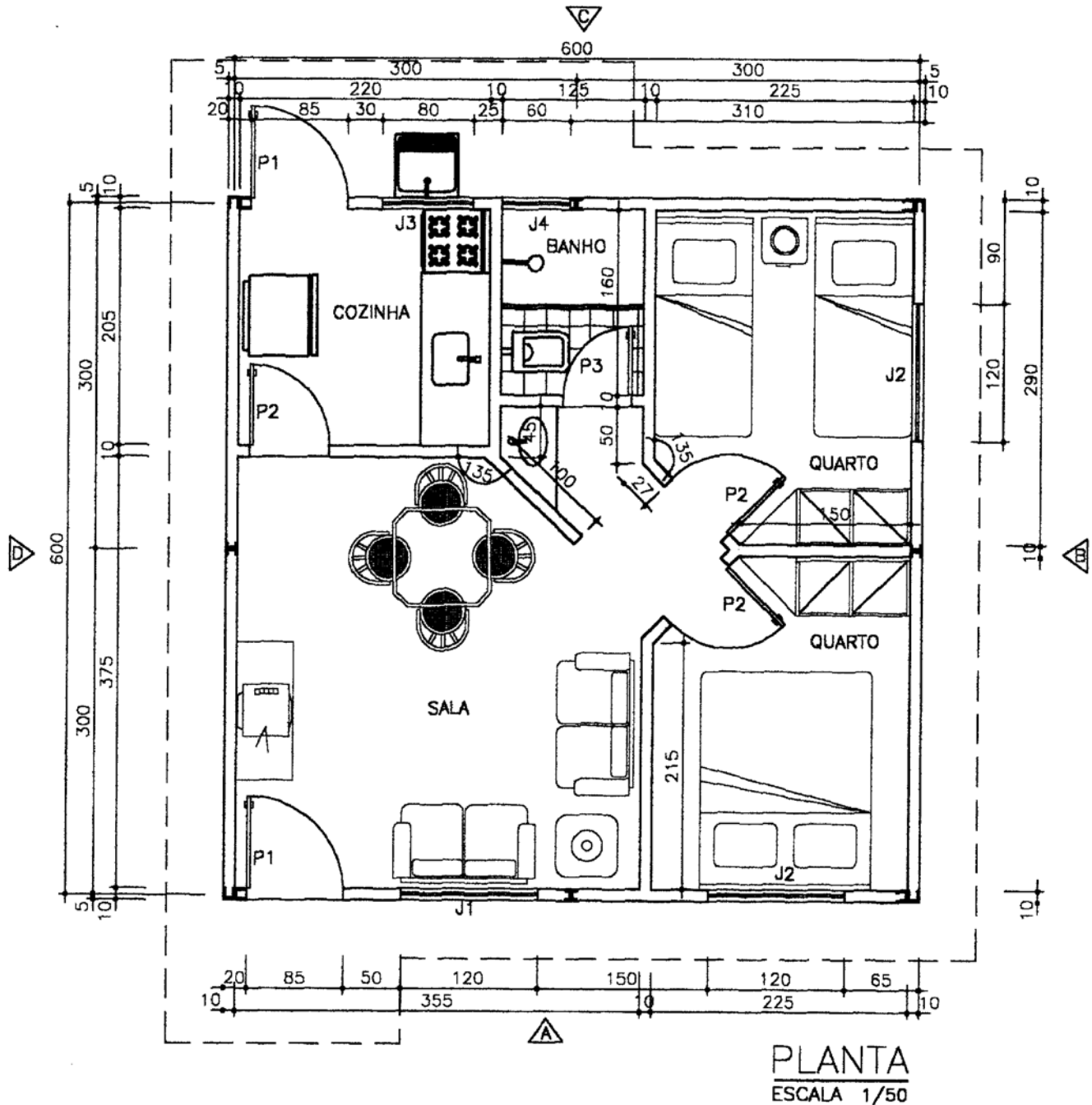
Figura 4 - Planta baixa da casa Usiteto. (Fonte: Usiminas, 2001).
