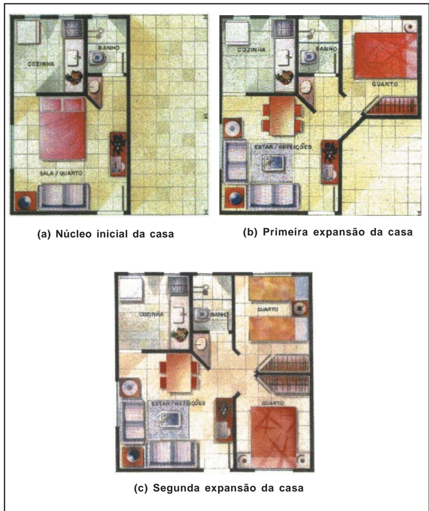
Figura 3 - Módulos da casa Usiteto. (Fonte: Usiminas, 2001).
