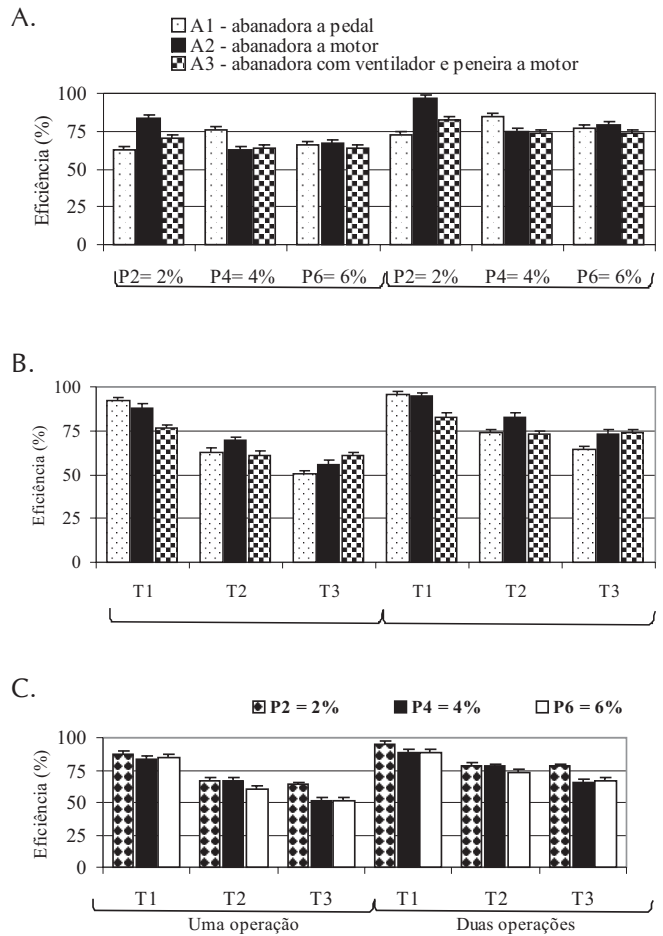
Figura 2. Eficiência de limpeza do arroz, proporcionada por uma ou por duas operações de diferentes abanadoras, (A) em função da porcentagem de impureza nas sementes, (B) da taxa de alimentação das máquinas e (C) da interação de percentual de impureza nas sementes com taxa de alimentação de sementes nas máquinas
