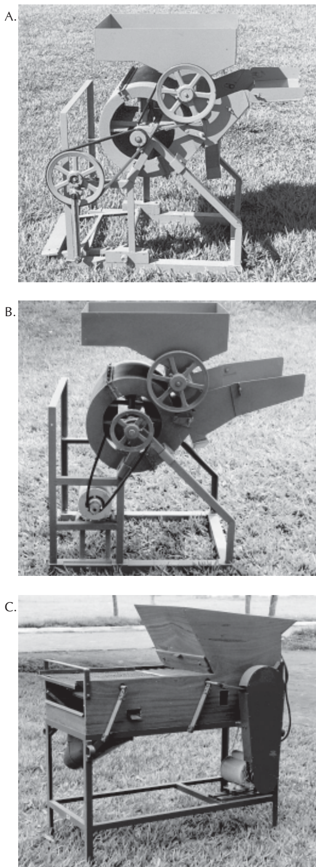
Figura 1. Abanadora de sementes com ventilador acionado a pedal: (A), com ventilador acionado a motor; (B) e com ventilador e peneira acionados a motor (C)
