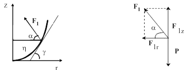
Figura 1 - (a) Vista lateral del movimiento de rotación de un fluido. (b) Esquema de las fuerzas actuando a distancia r_1 del eje de rotación.
