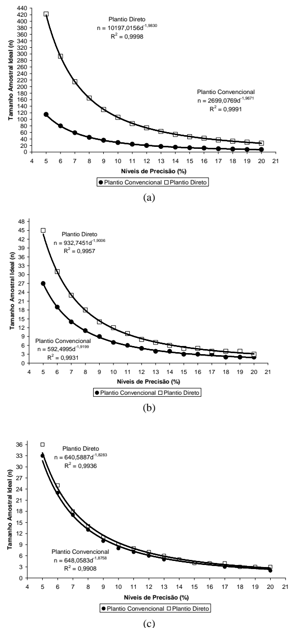
Figura 2. Relação entre o tamanho ideal amostral e o nível de precisão em torno da média para estimar os parâmetros: a) patinagem (%), b) capacidade de campo teórica ( m^2 s^{-1} ), c) capacidade de campo efetiva ( m^2 s^{-1} ).
