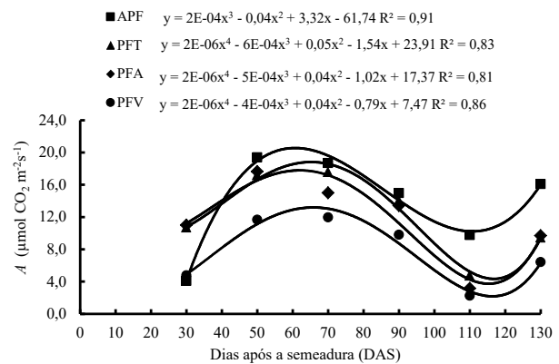
FIGURA 3: Valores médios da taxa de assimilação de CO 2 (A, μmol CO 2 m -2 s -1 ) de plantas de [ Peltophorum dubium (Spreng.) Taub.], submetidas a diferentes qualidades de luminosidade: Em que: APF: ausência de protetor físico; PFT: protetor físico transparente; PFA: protetor físico azul; PFV: protetor físico vermelho.
