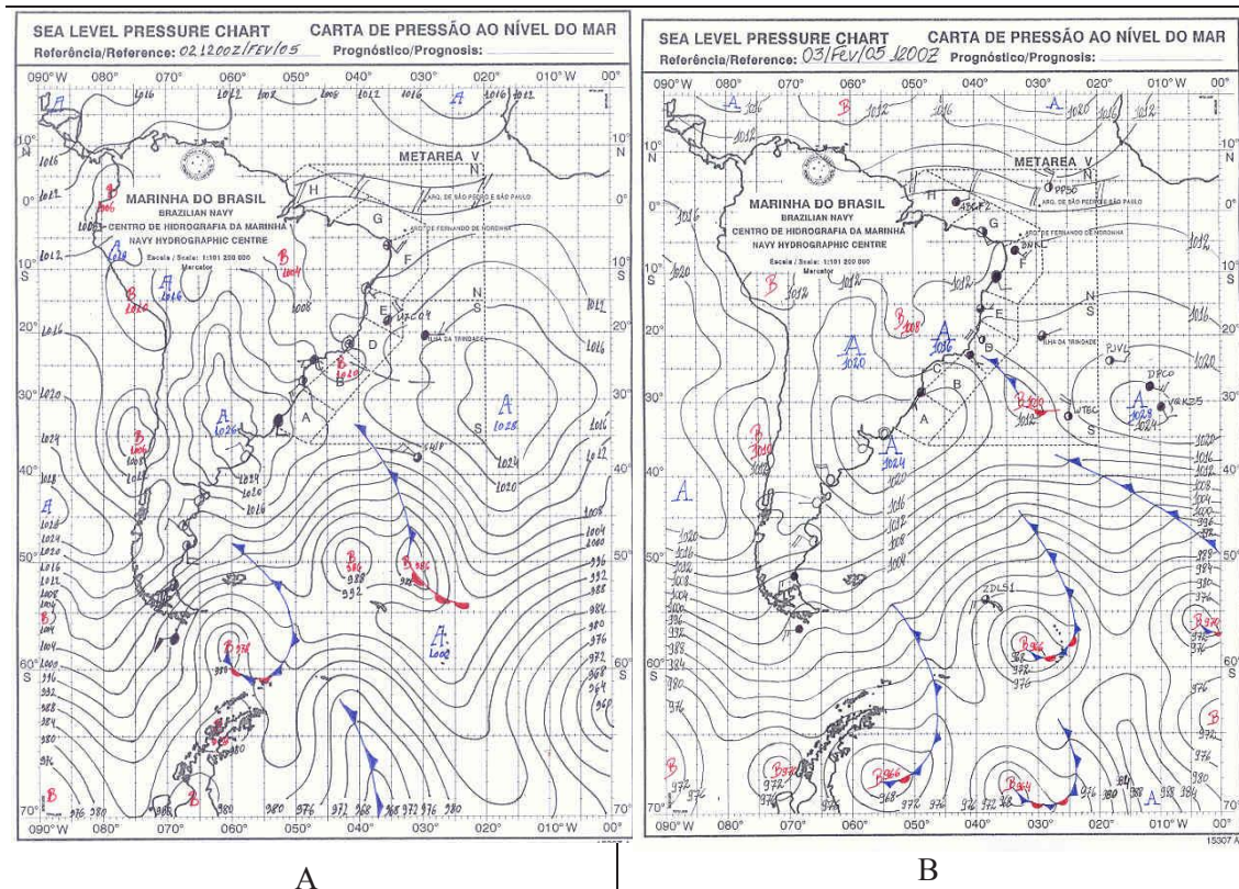
Figura 6 – As cartas A e B mostram as condições sinóticas nos dias 02 e 03 de fevereiro de 2005. No dia 02, a mPa avançou pelo interior do continente com 1026hPa; para o dia 03, ela se desintencificou e a pressão caiu para 1024hPa, e verificou-se um ligeiro deslocamento para o leste.
