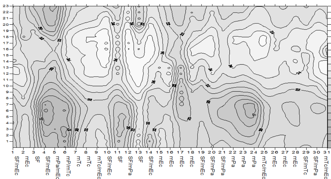
Figura 4 – Painel t mporo-espacial com as termoisopletas para o m s de janeiro de 2009 para Campo Mour o. Na abscissa, l e-se os dias do m s e os sistemas atmosf ricos, e na ordenada, as horas do dia. A mPa atuou integralmente na regi o de Campo Mour o nos dias 22, 23 e 24. Nesse per odo, a temperatura m nima foi de 17,0 C e a m xima 28,0  (Instituto Tecnol gico Simepar  2012).
