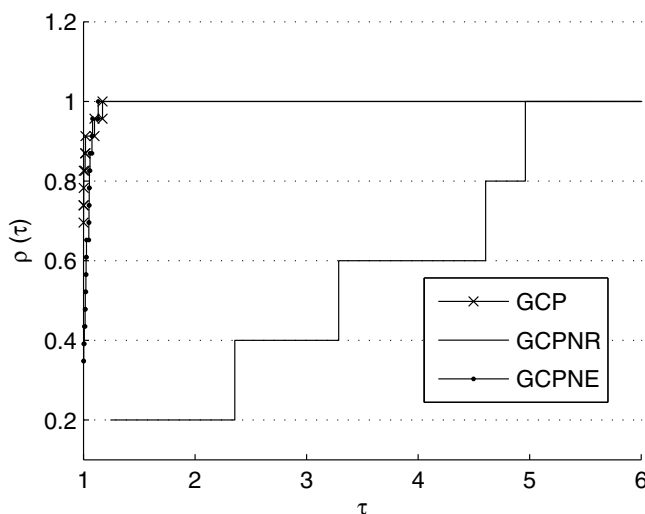
Figura 3: GCP, GCPNR e GCPNE – Perfil de desempenho: Tempo de Processamento.
