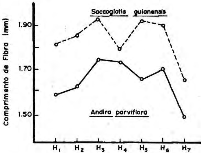
Fig. 8 - Média da variação radial do comprimento das fibras em diferentes alturas ao longo do tronco das espécies Saccoglottis guianensis e Andira parviflora .
