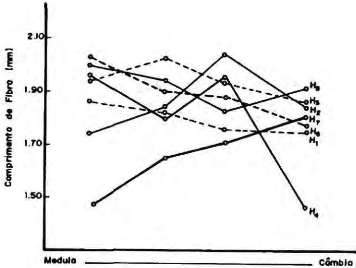
Fig. 3 - Variação radial (medula-câmbio) do comprimento das fibras em diferentes alturas do tronco em Saccoglottis guianensis .
