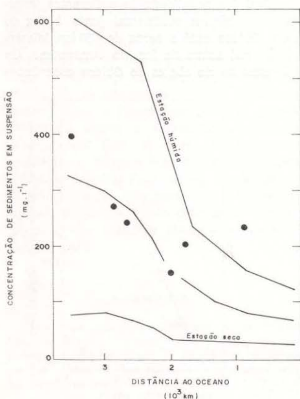
Fig. 2 — Concentrações de sedimentos em suspensão no curso principal do rio Amazonas. As linhas "a cheio" representam as concentrações indicadas por Gibbs (1967) para as estações úmidas, intermédias e secas. Os círculos negros representam as concentrações de material sólido em suspensão apresentadas na Tabela 1.
