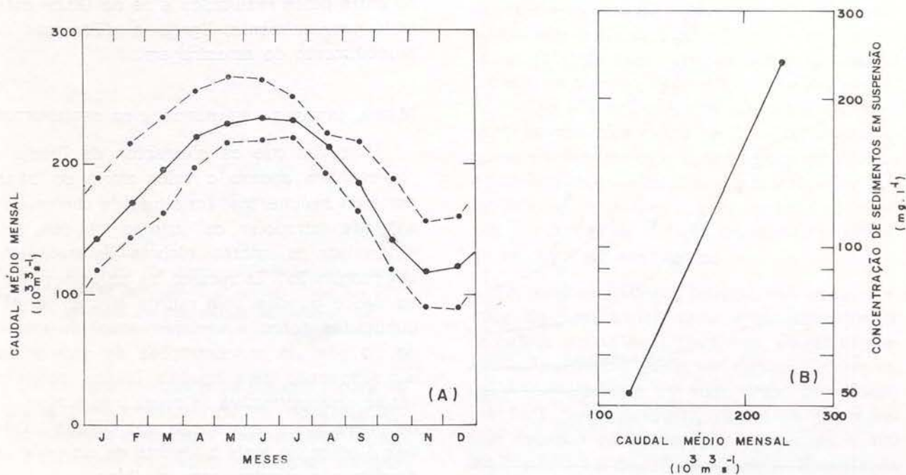
Fig. 3 — A) Caudais médios mensais do rio Amazonas em Óbidos, 1971-1975. Os máximos e mínimos dos caudais médios mensais são representados pelas linhas "a tracejado"; os valores médios são indicados pela linha "a cheio". Note-se que o máximo caudal médio mensal, para o período de quatro anos, é unicamente 3 vezes maior que o mínimo. B) Relação, admitida, entre a concentração média mensal de sedimentos em suspensão e caudal médio mensal em Óbidos.
