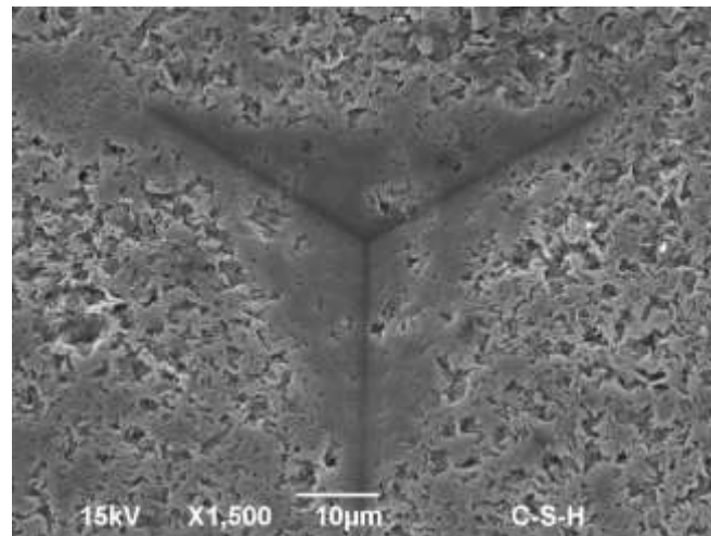
Figura 9 - Matriz Ca/Si 2,1 / Indentação 2 (14,2 GPa a 2 mN)
