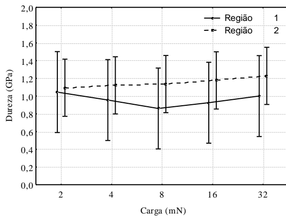
Figura 3 - Dureza do C-S-H com relações Ca/Si de 0,7 (a) e 2,1 (b)
