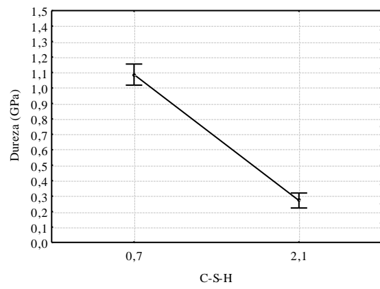
Figura 4 - Efeito da relação Ca/Si no módulo de elasticidade (a) e na dureza (b)
