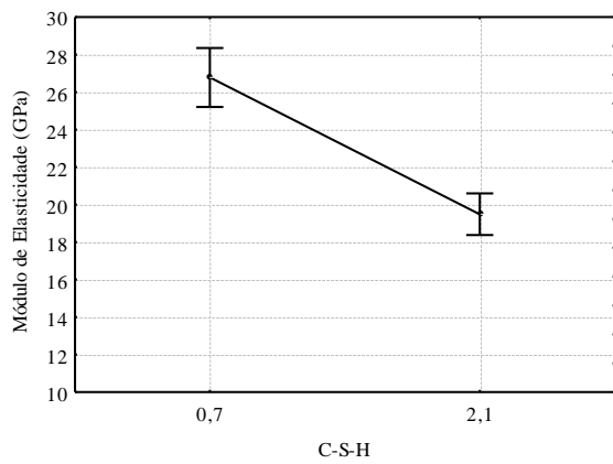
Figura 4 - Efeito da relação Ca/Si no módulo de elasticidade (a) e na dureza (b)
