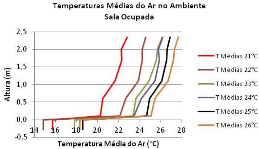
Figura 13 - Perfis de temperatura do ar (ambiente ocupado)
