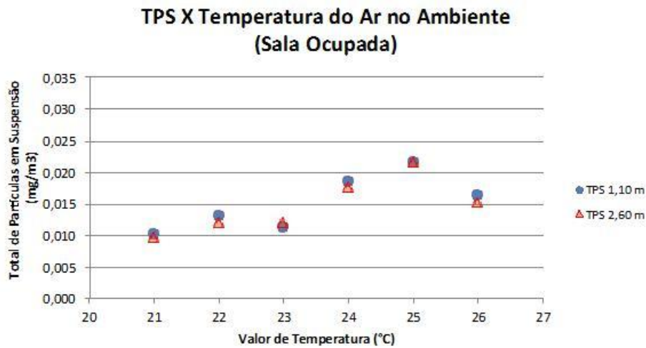
Figura 8 - TPS X Temperatura do ar: ambiente ocupado
