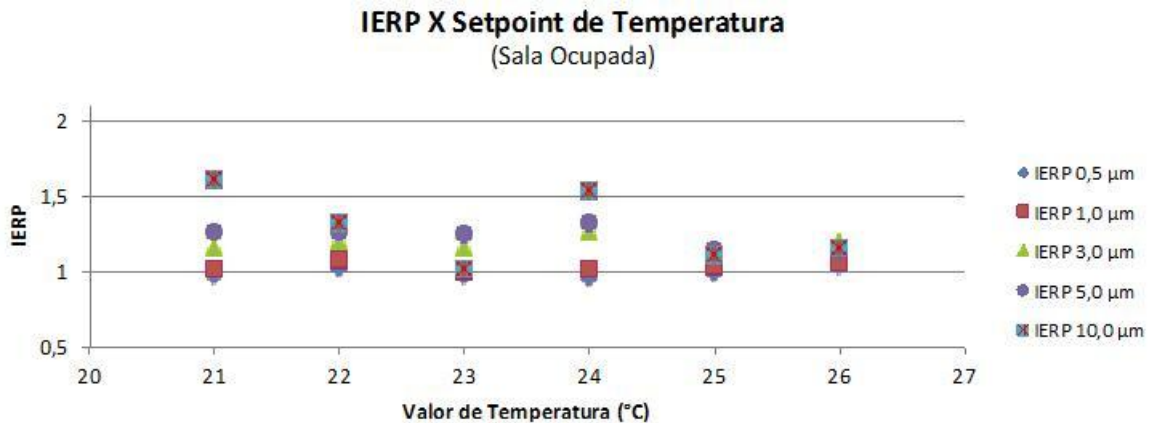
Figura 15 - IERP por tamanho de partícula X valor de temperatura do ar (ambiente ocupado)
