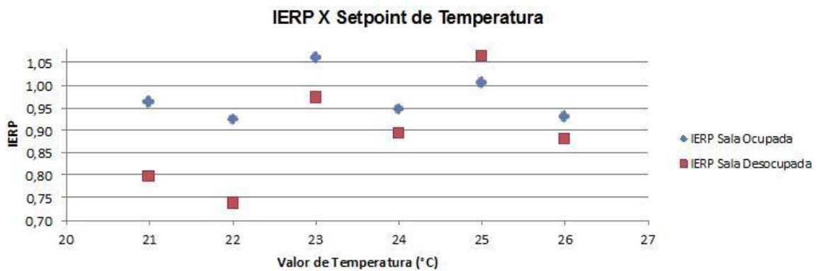
Figura 12 - IERP X Valores de temperatura do ar (ambiente ocupado e desocupado)
