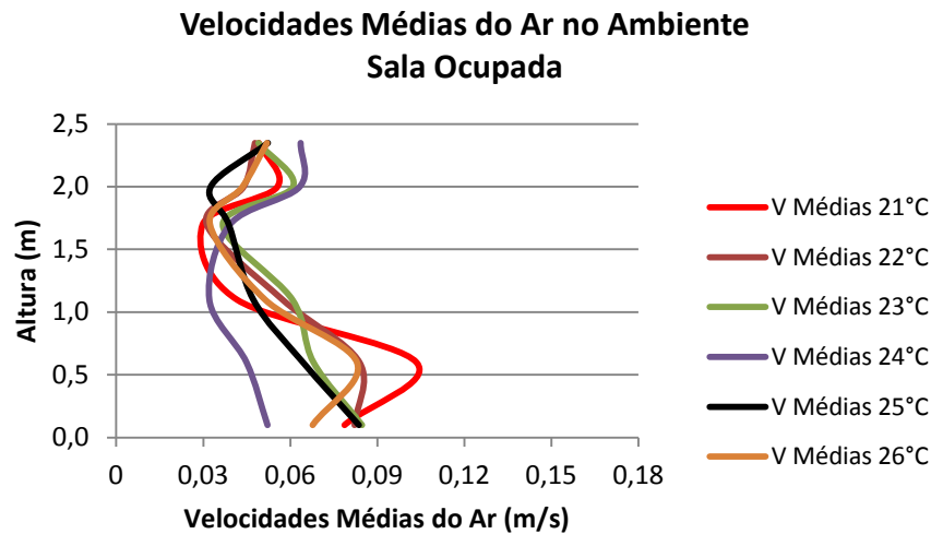
Figura 7 - Perfis de velocidade do ar: ambiente ocupado (1ª parte do estudo)
