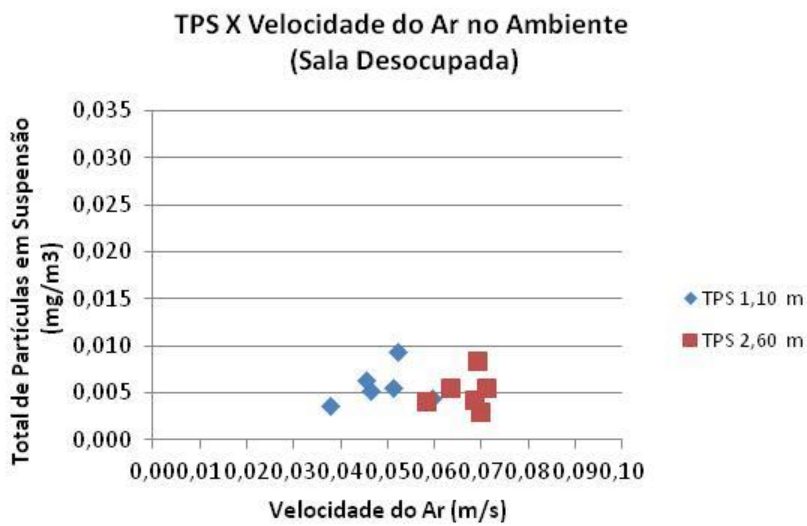
Figura 11 - TPS X Velocidade do ar: ambiente desocupado
