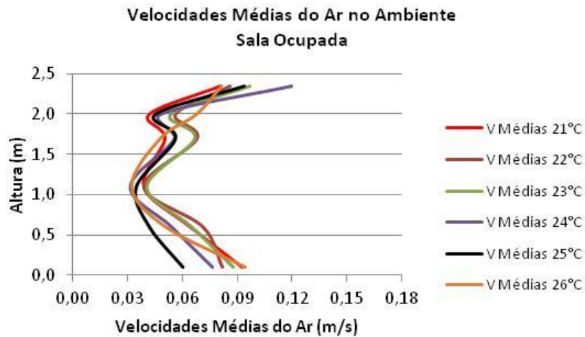
Figura 14 - Perfis de velocidade do ar (ambiente ocupado)
