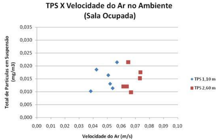
Figura 10 - TPS X Velocidade do ar: ambiente ocupado
