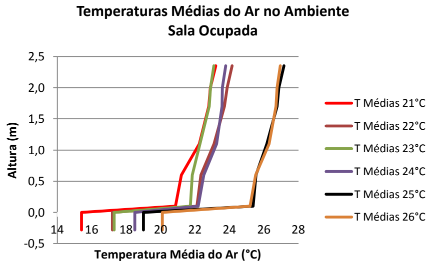
Figura 6 - Perfis de temperatura do ar: ambiente ocupado (1ª parte do estudo)
