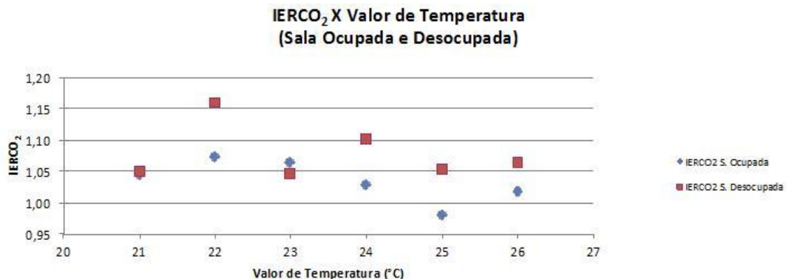
Figura 16 - IERCO 2 X Valor de temperatura do ar (ambiente ocupado e desocupado)
