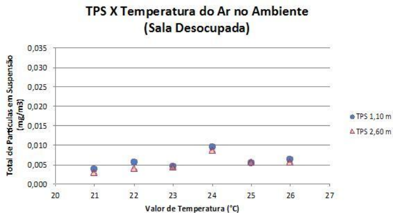
Figura 9 - TPS X Temperatura do ar: ambiente desocupado
