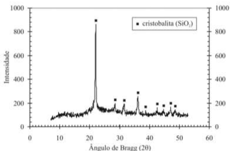
Figura 1 - Difratograma de raios X da cinza da casca de arroz - difratômetro Rigaku Miniflex com tubo de Cu-K \alpha
