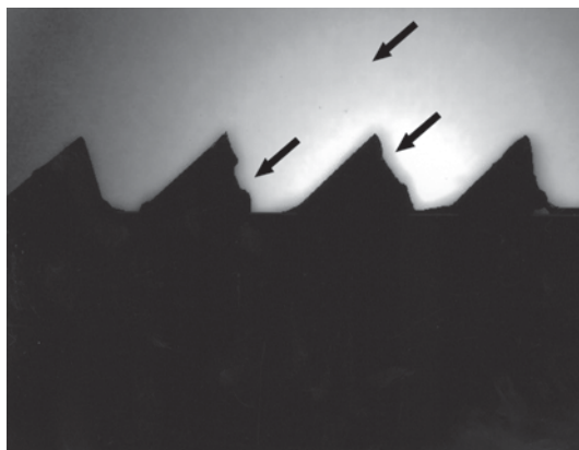
Figura 8 – Detalhe da projeção de perfil de parafuso ósseo, apresentando duas roscas adjacentes com irregularidades em sua superfície (setas).
