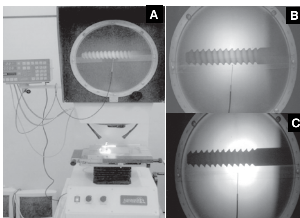
Figura 7 – Avaliação metrológica dos parafusos. Projetor de perfil (A). B - Imagem obtida no modo episcopia e, C - imagem obtida no modo diascopeia.
