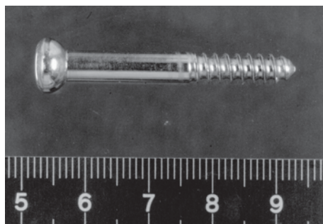
Figura 6 - Parafuso metálico de rosca rasa tipo vástago.
