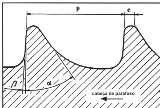
Figura 4 - Ilustração dos ângulos \alpha ( 35^\circ ) e \beta ( 3^\circ ), do passo ( p = 1,75 mm) e do comprimento do ápice da rosca ( e = 0,1 mm). Fonte: ABNT (1996).
