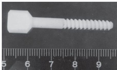
Figura 3 - Parafuso ósseo obtido.
